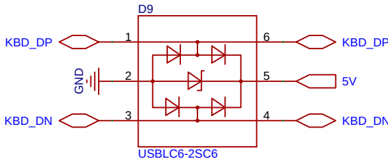
ESD Suppressor
